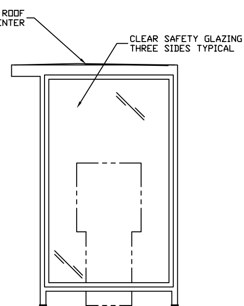
E4 ELEVATION
