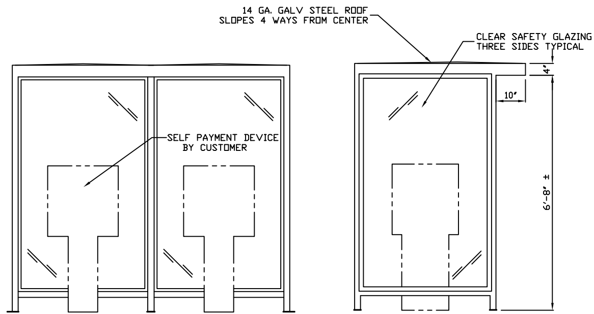
E1 ELEVATION
