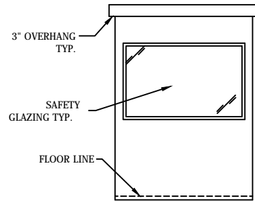
E2 ELEVATION
