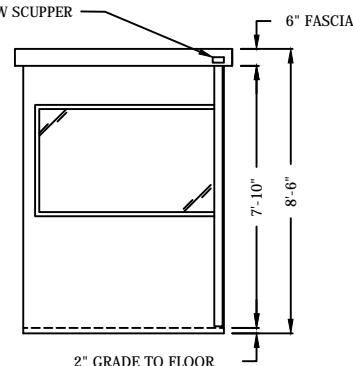
E4 ELEVATION
