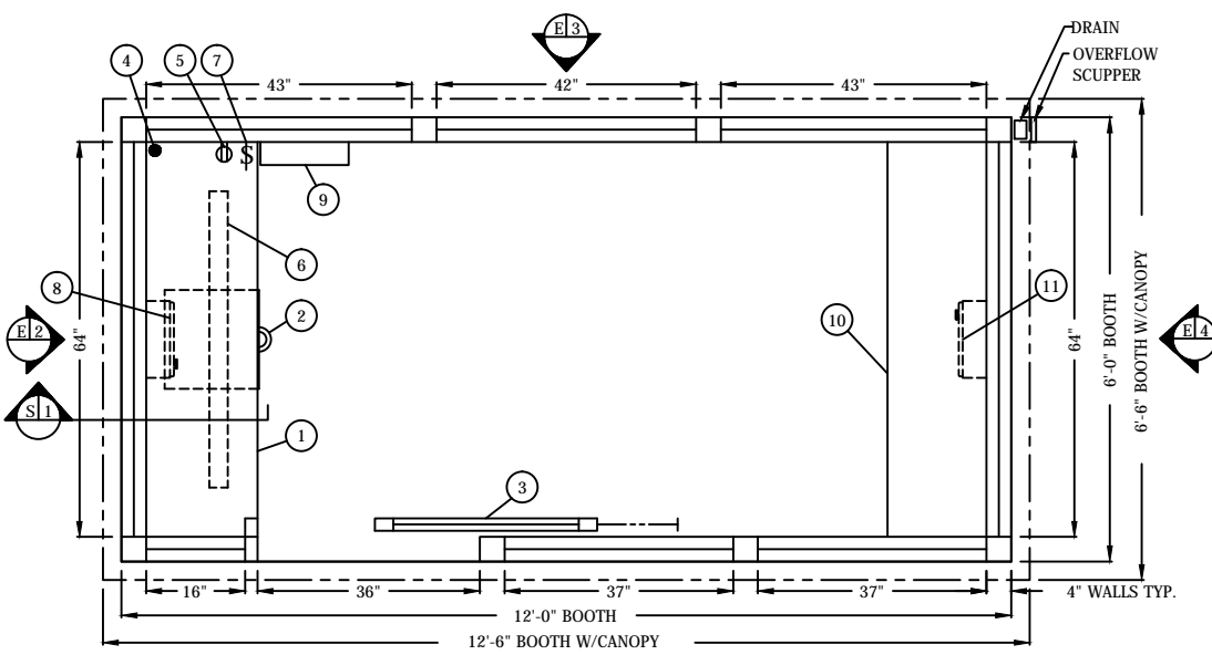
E1 PLAN VIEW
