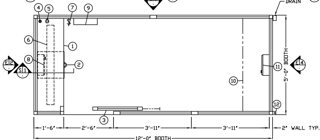
E1 PLAN VIEW
