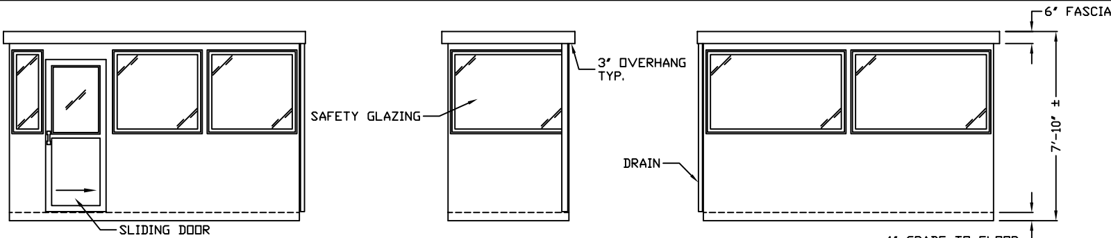
E1 ELEVATION
